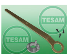
Klucz do blokowania koła pasowego wału Mercedes M271
