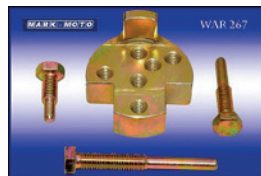
Przyrząd do demontażu i montażu pasków wielorowkowych Stretch
