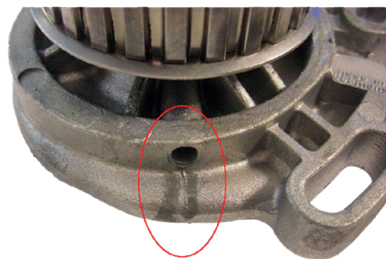
Widoczny wyciek płynu z otworu technologicznego pompy cieczy
